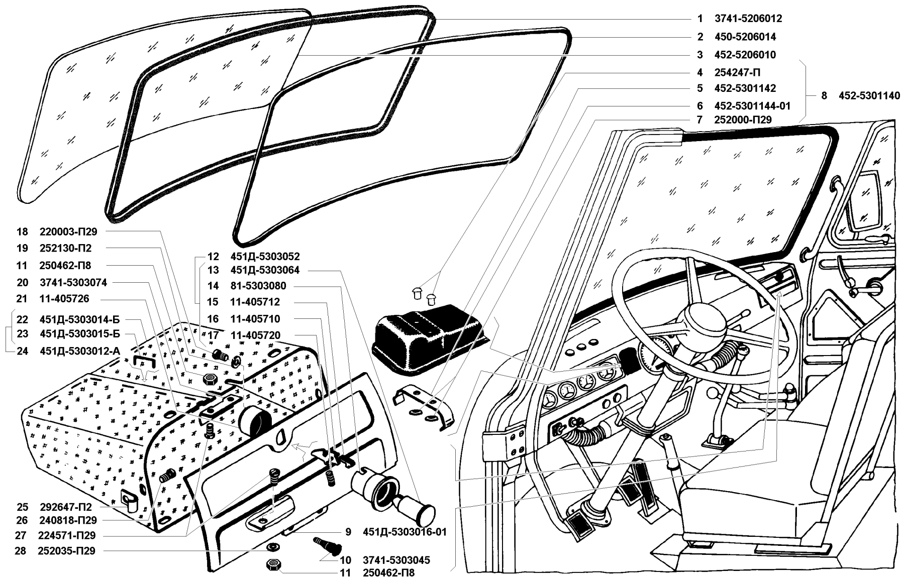
Рис. 125. Стекло, уплотнители ветрового окна (5206,) передок (5301), ящик вещевого (5303) Fig. 125. Glass, windshield weatherstrips (5206), body front (5301), glove box (5303)
